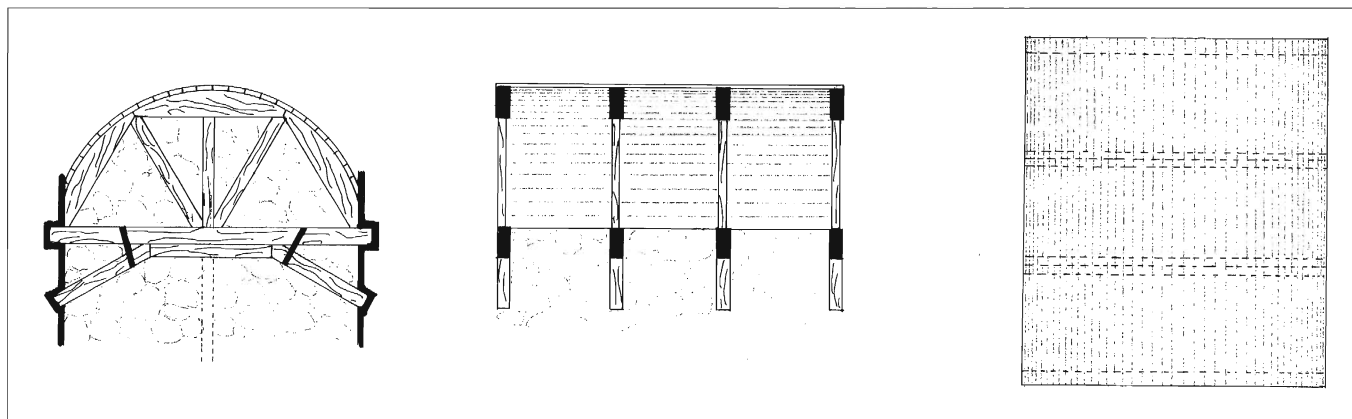
Cintra per a voltes de canó (torres de planta quadrada)
