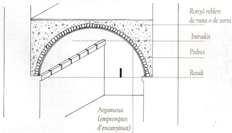
La volta: parts i materials utilitzats
