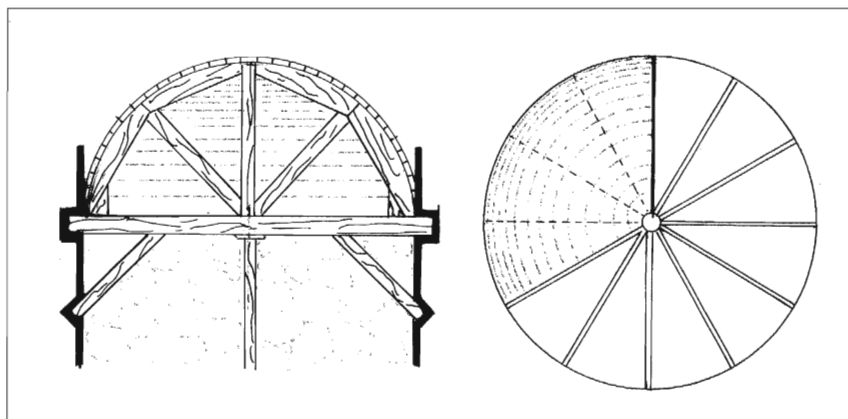
Cintra per a voltes esfèriques (torres de planta rodona)
