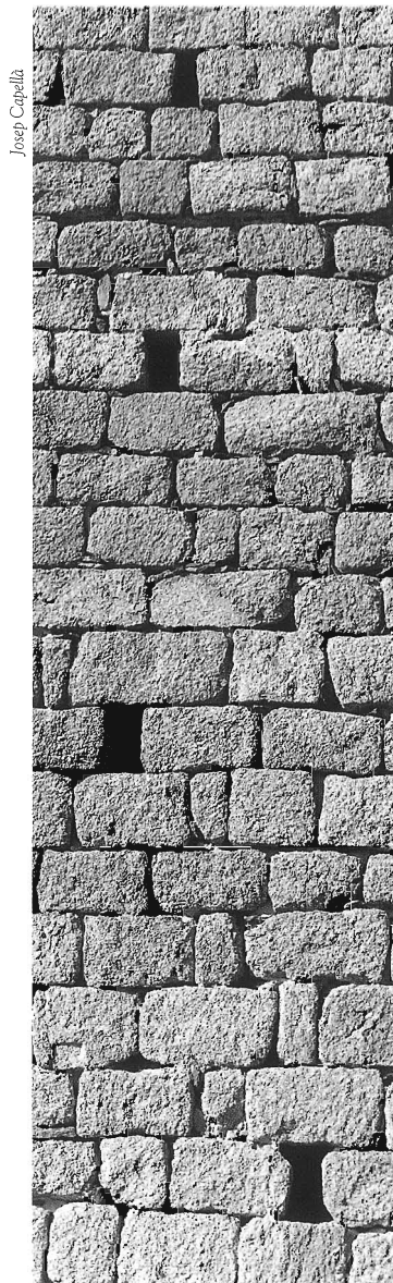
Els murs de la torre Simona presenten encara els forats deixats per les bastides utilitzades a la seva construcció. Alguns d'aquests forats es van aprofitar per ser utilitzats com-espitlleres
