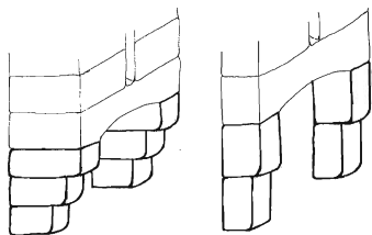
Croquis d'una mènula i d'una cartel·la
