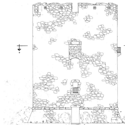
Alçat cara tramuntana
