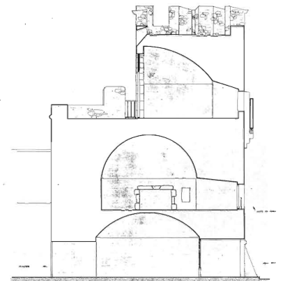
Secció A-A'
