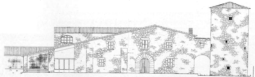
Alçat cara migdia
