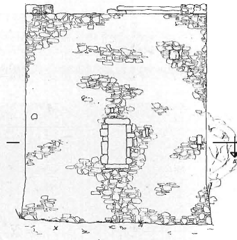
Alçat cara migdia
