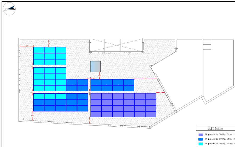
Figura 12. Distribució panells fotovoltaics de la instal·lació
