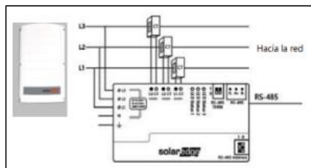
Figura 11. Esquema de connexió de l'equip de monitorització i toroidals
