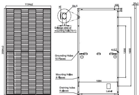
Figura 3. Panell fotovoltaic
