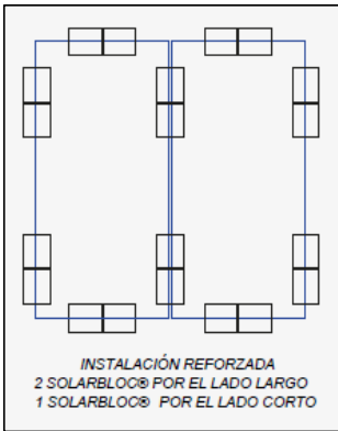
Figura 6. Configuració Blocs de formigó a instal·lar
