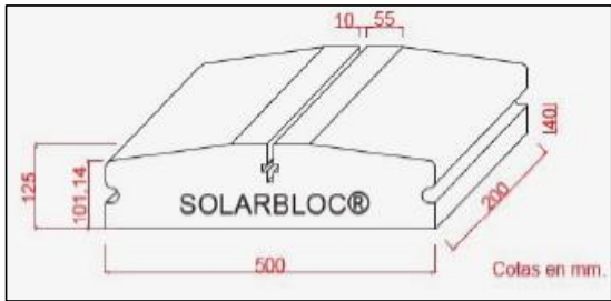
Figura 5. Mesures Bloc de formigó
