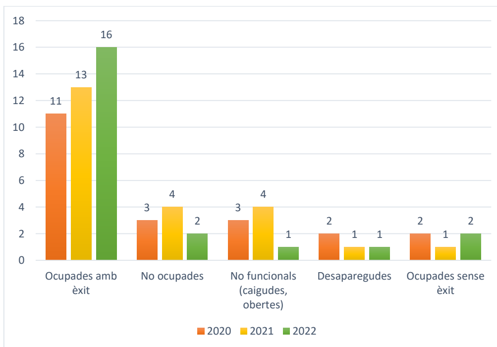
Gràfic 1. Gràfic resum de la ocupació de les caixes niu per a ocells, la temporada de 2020.
