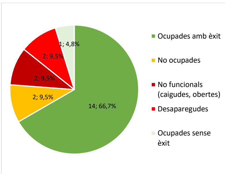
Gràfic 3. Gràfic resum de la ocupació de les caixes niu per a ocells, la temporada de 2021.
