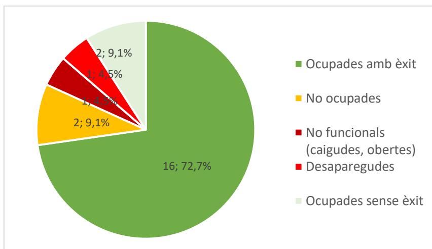
Gràfic 4. Gràfic resum de la ocupació de les caixes niu per a ocells, la temporada de 2022.
