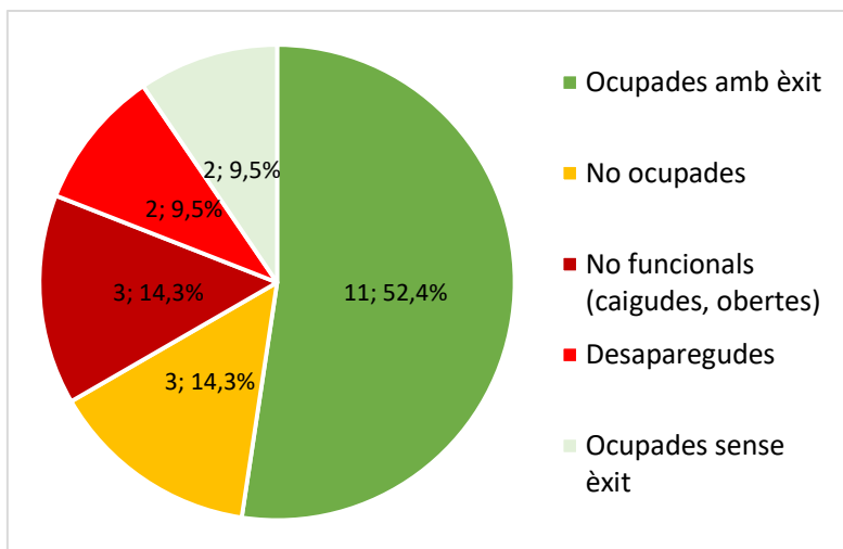
Gràfic 2. Gràfic resum de la ocupació de les caixes niu per a ocells, la temporada de 2020.
